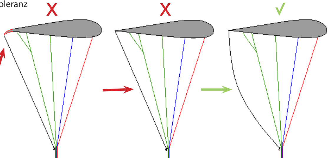
Toleranz
